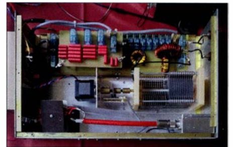
Bild 3: Blick in den von DL4JAL aufgebauten Antennenkoppler nebst Symmetrierbalun nach DG0SA Foto: DL2AVH
