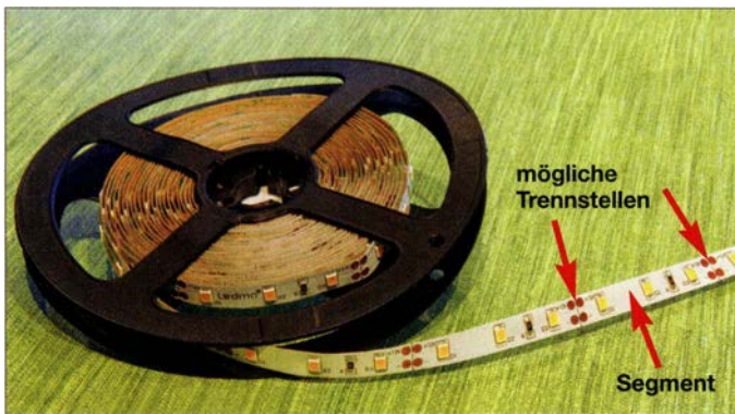
Bild 1: Dieser 5 m lange LED-Streifen mit 300 LEDs besteht aus insgesamt 100 Segmenten, sodass sich der Streifen bei Bedarf an nahezu beliebiger Stelle kürzen lässt.
