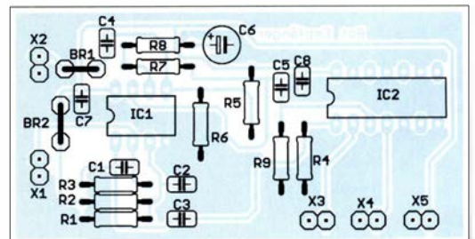
Bild 10: Bestückungsplan der Platine des Senders; Abmessungen 27,6 mm x 32,7 mm, M 1:1
