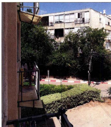
Ganz unscheinbar neben den Wäscheleinen im ersten Stock: 4X1GAs 70-MHz-Antenne, der Aluminiumrahmen des Fensters mag als Reflektor Richtung Nordwest gewirkt haben. Foto: 4X1GA
