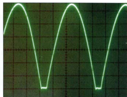
Bild 18: Gemessener zeitlicher Verlauf der Ausgangsspannung des Pulsweitenmodulators bei der Einstellung PWM_{\min} = 100
