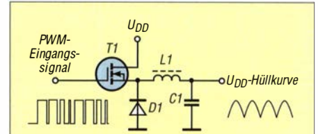
Bild 3: Ansteuerung des Abwärtswandlers mit dem PWM-Signal aus dem Hermes-Transceiver
