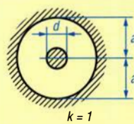
Bild 3: Rundes Rohr
