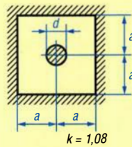
Bild 4: Quadratisches Rohr
