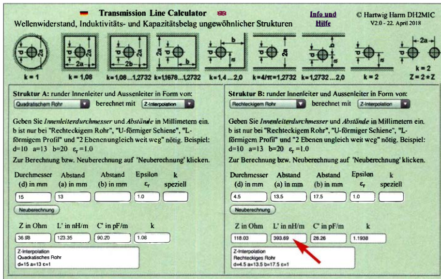
Bild 13: Screenshot des Programms Transmission Line Calculator ; in den Rechenblättern sind links die Berechnung einer koaxialen Transformationsleitung mit quadratischem Außenleiter zur \lambda/4 -Transformation von 25 \Omega auf 50 \Omega sowie rechts die Bestimmung von Wellenwiderstand, Induktivitäts- und Kapazitätsbelag eines 4,5 mm dicken Leiters in einer rechteckförmigen Außenleiterstruktur zu sehen. Foto, Screenshot: DH2MIC
