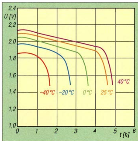
Bild 8: Verlauf der Zellenspannung eines Bleiakkulators bei 0,1 I_1 Entladestrom und verschiedenen Temperaturen Daten: [10]
