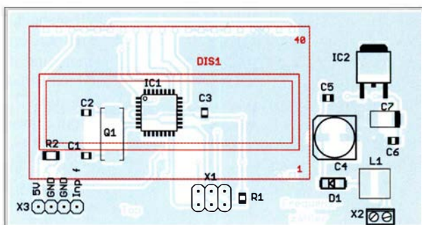
Bild 8: Bestückungsplan der Platine des Frequenzzählers mit dem Display auf der Unterseite; Abmessungen 82,5 mm x 42,8 mm, M 1:1
