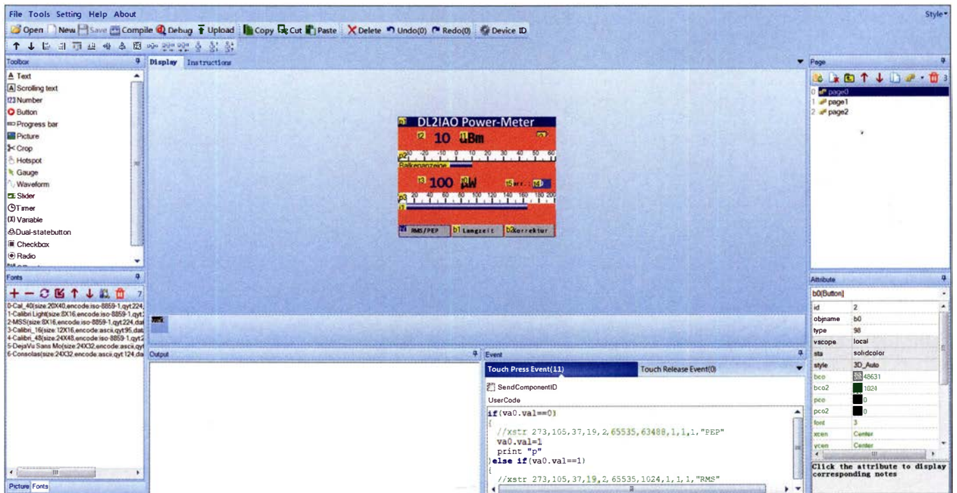
Bild 7: Grafische Programmieroberfläche für Nextion-Displays, hier mit der ersten Seite des HF-Leistungsmessgeräts (page 0); links befinden sich die Toolbox und die Übersicht über die geladenen Schriftarten, unten sind Ausgabe- und Befehlsfenster, rechts Seiten- und Eigenschaftfenster zu sehen.
