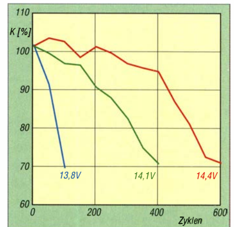
Bild 6: Die Lebensdauer eines Bleigel-Akkumulators ist bei zu niedriger Ladenspannung stark reduziert. Daten: [5]
