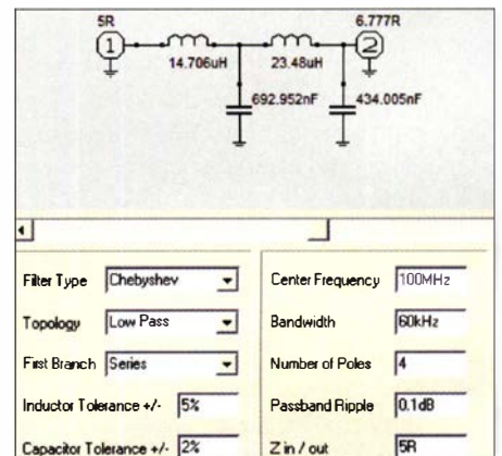
Bild 15: Ermittlung der Bauelementwerte für das Ausgangstiefpassfilter mittels RFSim99 (hier: PWM für 100-V-Endstufen)
