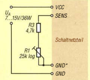
Bild 6: Zusatzschaltung zur Nutzung des Schaltnetzteils als einstellbare Spannungsquelle
