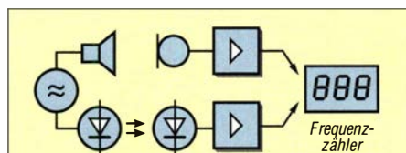
Bild 2: Der Dopplereffekt kann mit akustischen und mit optischen Signalen getestet werden.
