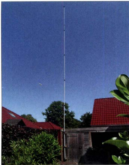
Bild 2: Dank 12 m Länge eignet sich die EFW lewis als Vertikalstrahler an einem GFK-Mast.
