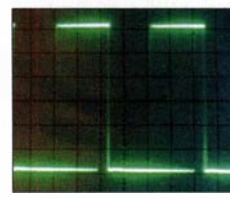
Bild 6: Oszillogramm der steilflankigen 12-V-PWM-Impulse am Ausgang des Eingangstreiber-schaltkreises
