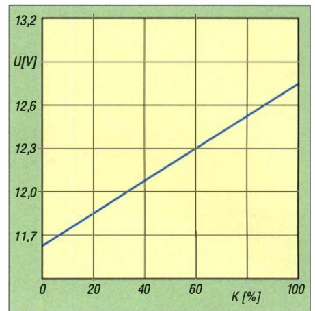
Bild 9: Der Zusammenhang zwischen Ruhe-spannung und Ladezustand eines Bleiakkulators. Daten: [10]
