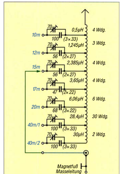
Bild 6: Schaltplan der Antenne; der ange deutete Innenleiter des Koaxialkabels zum Transceiver (blau) führt über das Aluminiumdrehteil an der Unterseite des Spulenkörpers auf die „Wanderleitung“ (grün) und von dort an den gewählten Spulenabgriff.
